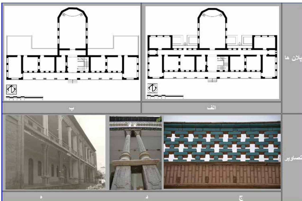
تصویر ۵. دبیرستان سعدی: الف) پلان طبقه همکف؛ ب) پلان طبقه اول (برداشت: نگارندگان؛ ج) جان پناه ساختمان؛ د) ستون‌های دوقلوه؛ ه) نمای جنوبی. عکس‌ها از مهران کاراحمدی؛ مأخذ تصویر ۵-۵: آرشیو موزه آموزش و پرورش.
