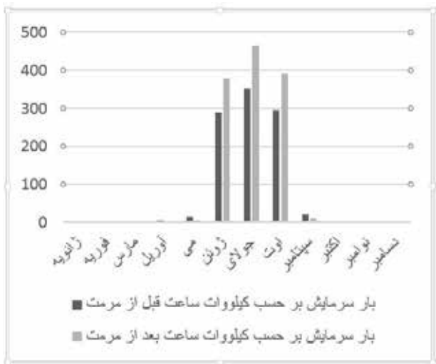
نمودار ۵. بار سرمایش اتاق دودری زیرزمین خانه علمی قبل و بعد از مرمت. مأخذ: نگارندگان.
