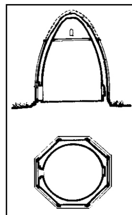
تصویر ۷. پلان و برش آرامگاه ملک اژدر در لاجین مأخذ: Qiyasi 1991
