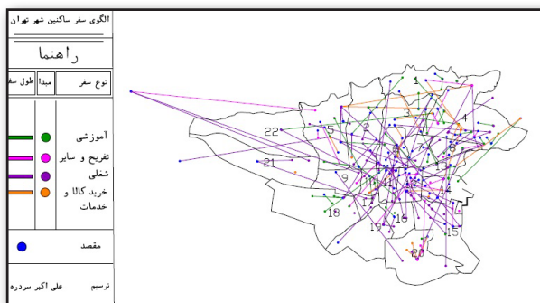
تصویر ۴. مبدأ و مقصد و فواصل سفر افراد حاضر در نمونه به تفکیک اهداف سفر. مأخذ: ترسیم نگارندگان با استفاده از اطلاعات شرکت مطالعات جامع حمل و نقل تهران، ۱۳۸۶. Fig. 4. The origin, destination and travel distance for sampled residents. Source: authors based on data provided by Tehran Comprehensive Transportation and Traffic Company (TCTTS), 2007.
