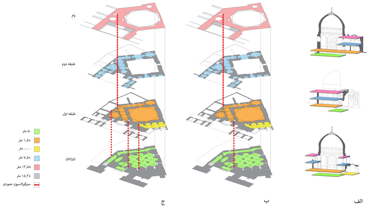
تصویر ۹. تحولات سیرکولاسیون عمودی بنا. الف: ترازهای ارتفاعی مختلف در برش‌های بنا؛ ب: سیرکولاسیون عمودی بنا در حال حاضر؛ ج: سیرکولاسیون عمودی بنا در گذشته؛ تصاویر مسدود شدن راه پله‌ها در مقایسه بخش ب و ج. مأخذ: نگارندگان.
