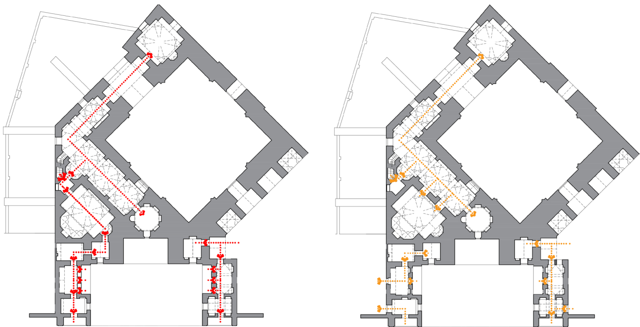
تصویر ۷. تحولات سیرکولاسیون طبقه دوم بنا در گذشته؛ چپ: سیرکولاسیون طبقه دوم بنا، اکنون. مأخذ: نگارندگان.
