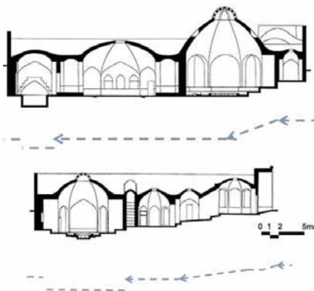
تصویر ۸. نمایش برش شیب کف در گرمابه تاریخی گلشن یزد. مأخذ: حاجی قاسمی، ۱۳۸۳.
