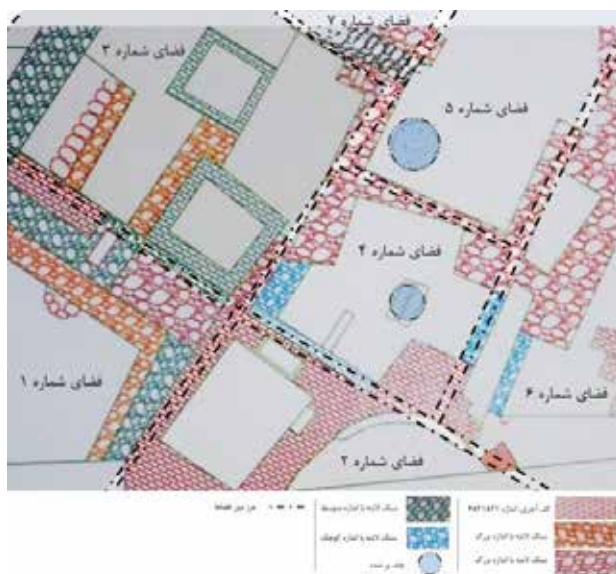
تصویر ۴. پلان فضابندی‌های درونی ساختار معماری مکشوف معروف به گرمابه ربع رشیدی. مأخذ: نگارندگان؛ بر اساس طرحی از روح‌انگیز، ۱۳۸۶.
