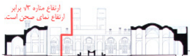
تصویر ۱۹. نمای شرقی صحن مسجد-مدرسه فیلسوف‌الدوله. مأخذ: حاجی قاسمی، ۱۳۷۷، ۱۳۱.
