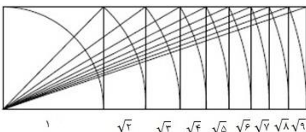
تصویر ۲. رسم مستطیل \sqrt{2} و گسترش آن. مأخذ: بوزجانی، ۱۳۷۶، ۱۲۵.
