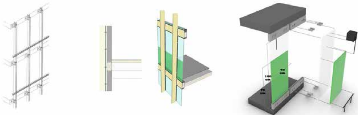
تصویر ۲. ابعاد مورد نظر، سازه پشتیبان و نحوه اتصال زیست‌رآکتور به نما. مأخذ: رضازاده، ۱۳۹۷.
