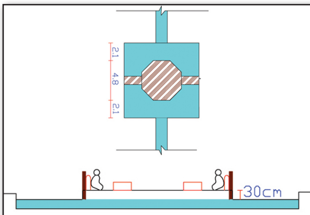
تصویر ۷. پلان و برش عرضی حوض دوم با تخت مشمن در وسط آن بنا به گفته‌های شاردن، مأخذ: نگارنده.
