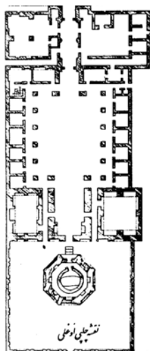
تصویر ۱۷. پلان خانقاه چلبی اوغلو مأخذ: مخلصی، ۱۳۶۹
