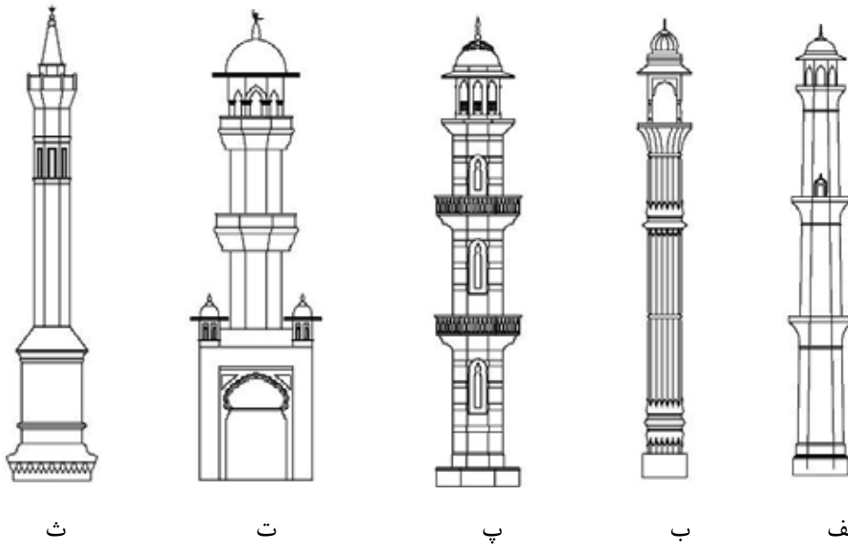
تصویر ۳. مناره‌ها الف) مسجد جامع دهلی ب) مسجد قاضی‌الدین خان، دهلی پ) مسجد جامک کوالامپور ت) مسجد کاپیتان کلینگ، پنانگ ث) مسجد ظهیر الورستار. مأخذ: نگارندگان.
